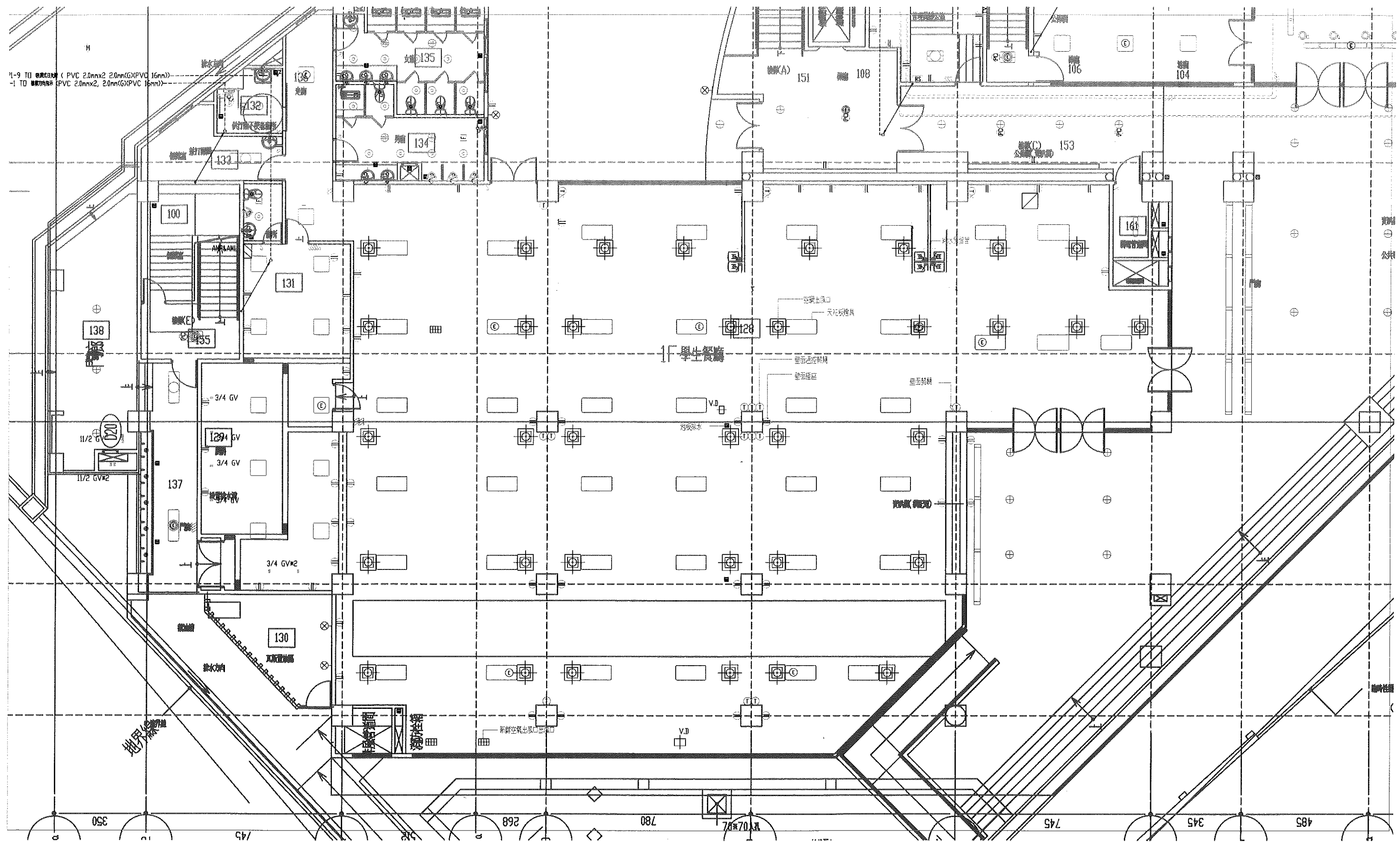
勤益學舍一樓學生餐廳設備配置示意圖
