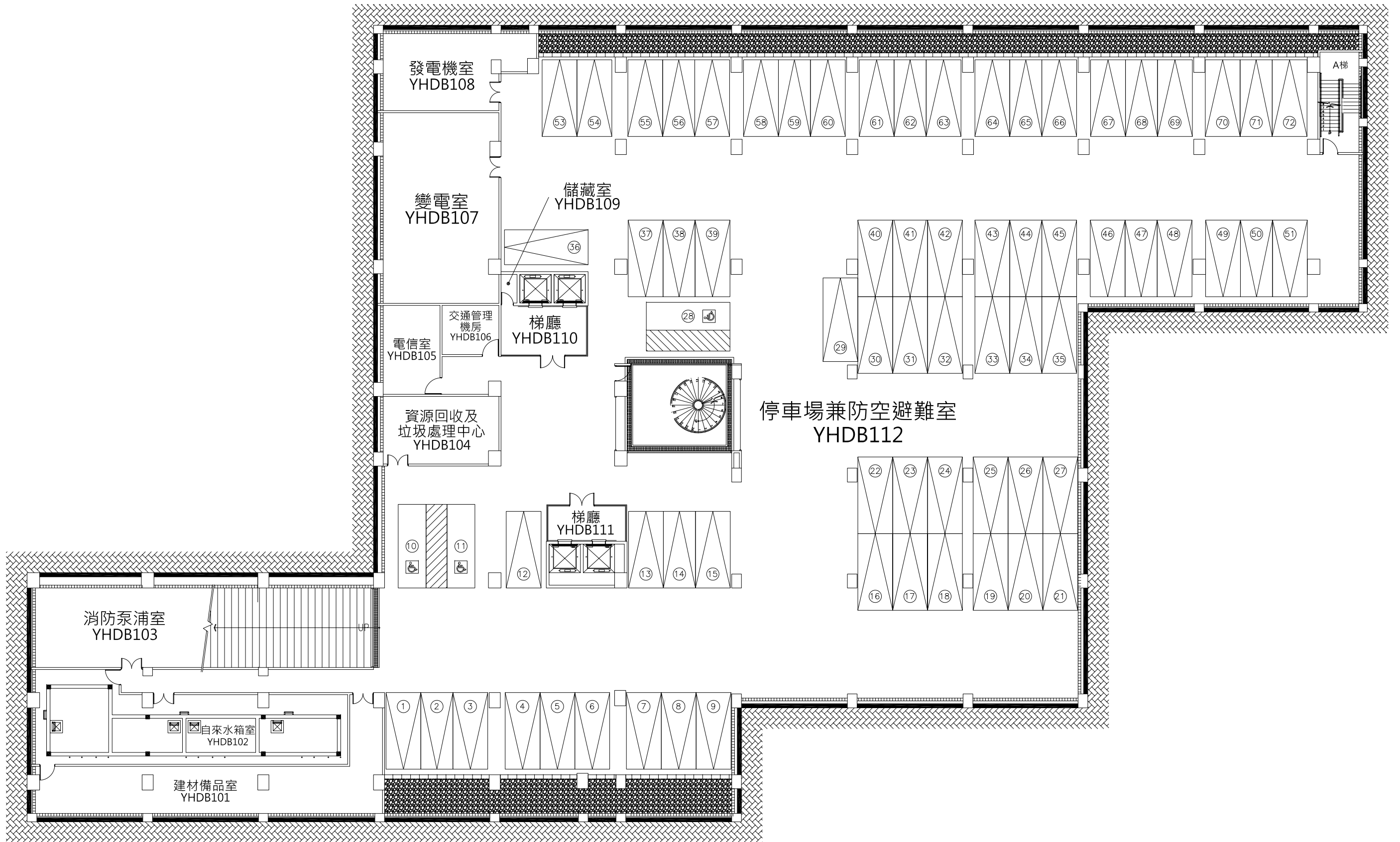
地下一層平面圖
