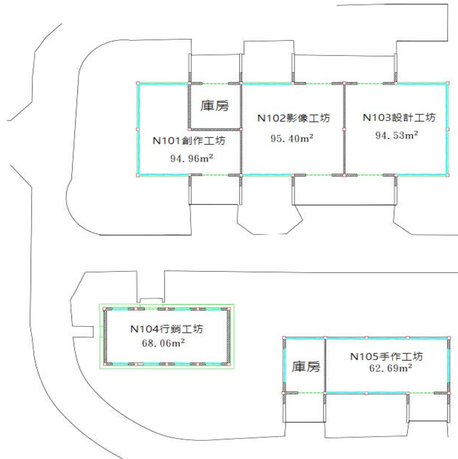
彈藥庫(勤益創作基地)平面圖
