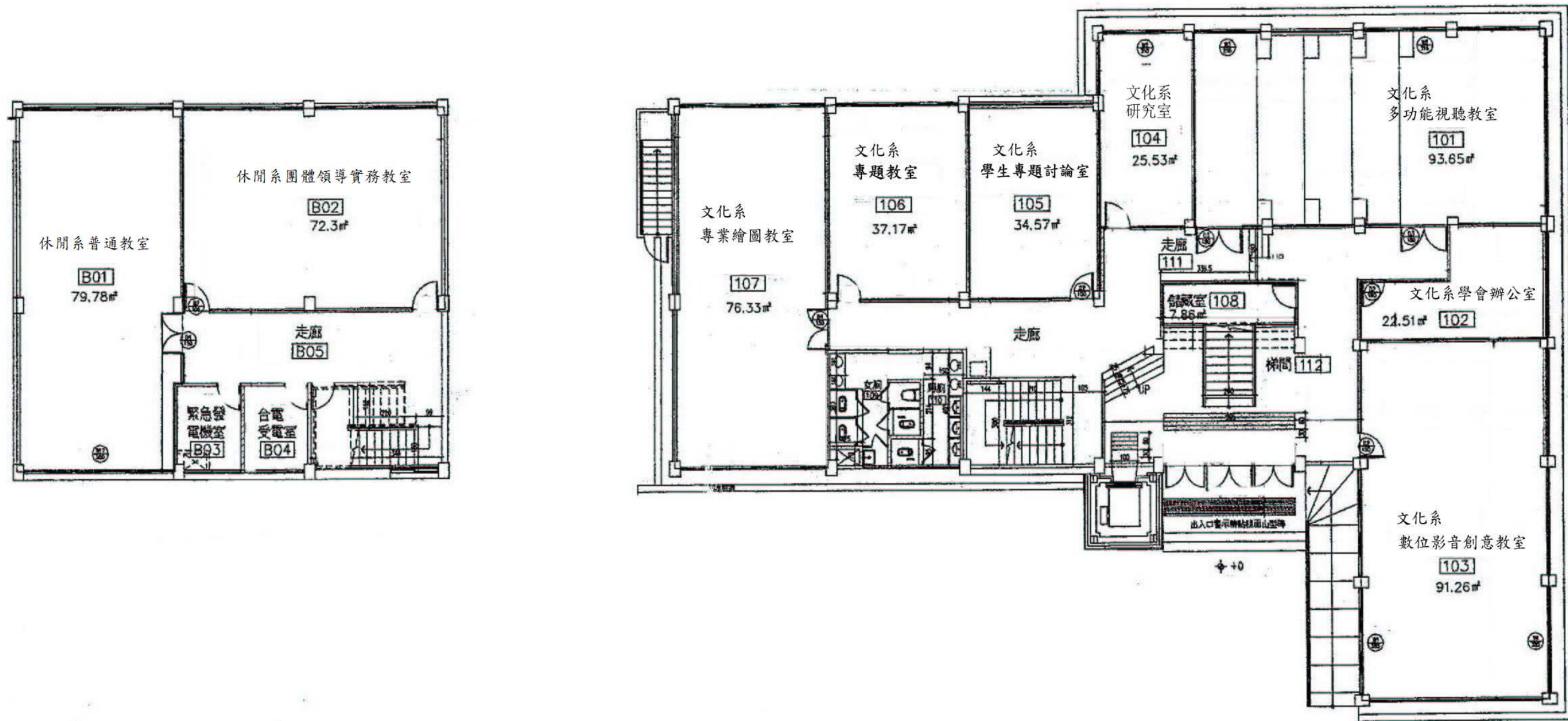
文化休閒館地下一樓及一樓平面圖
