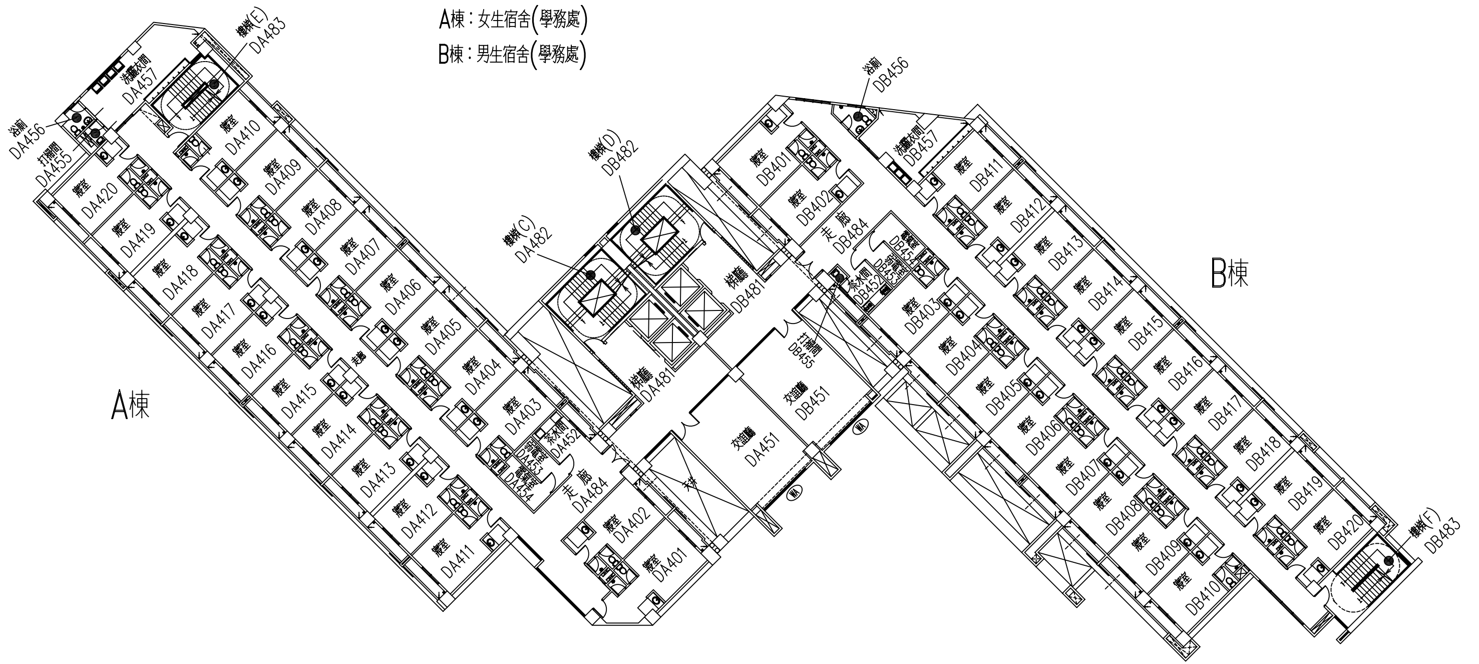
勤益學舍四樓平面圖
